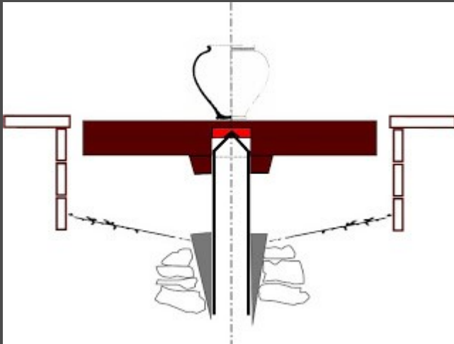
Schéma de fonctionnement d'un tour de potier, Pierre-Alain Capt ©2011
