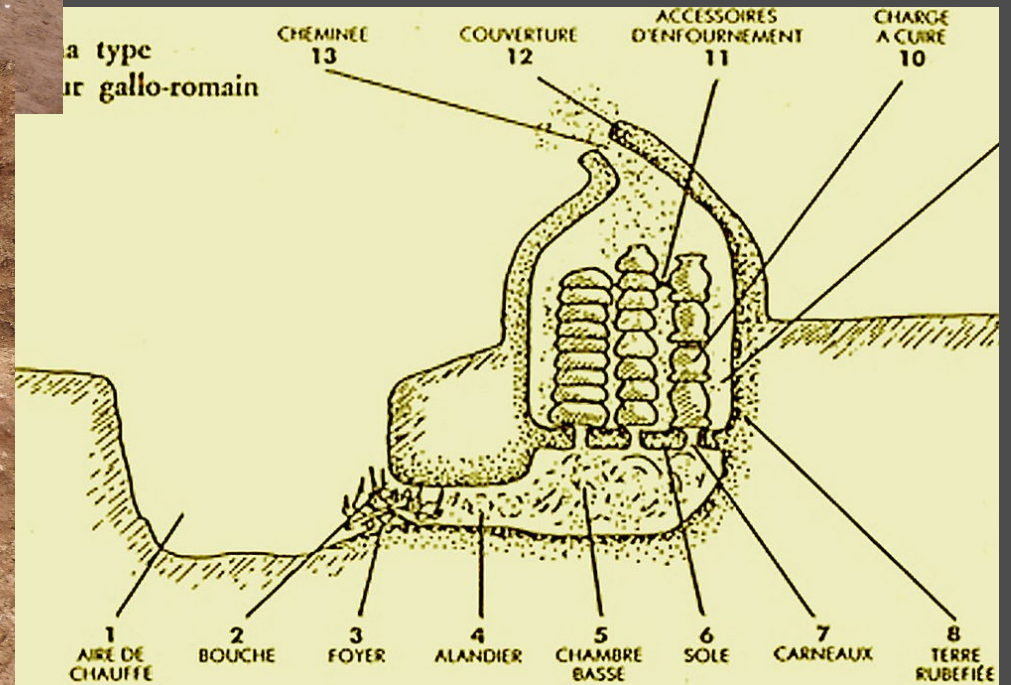
Exemple de restitution de four romain, Par JPS68 — Travail personnel, CC BY-SA 4.0, https://commons.wikimedia.org/w/index.php?curid=38064318
